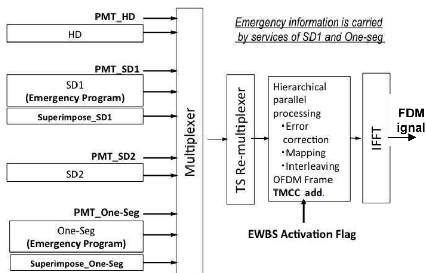
Figura 2 – Ejemplo de operación de transmisión del EWBS
